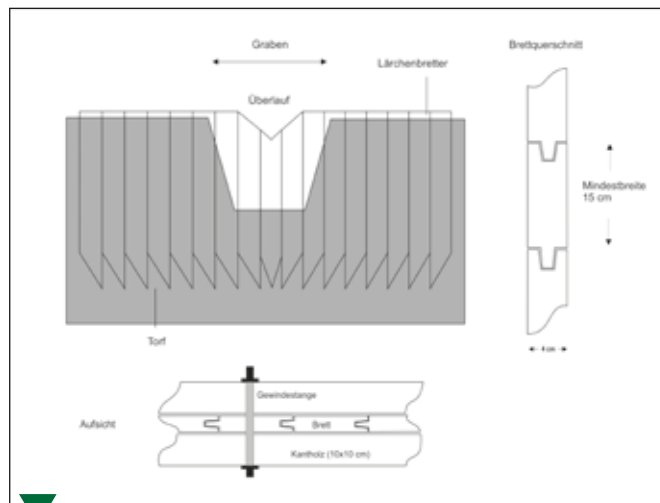
Schematische Darstellung eines Damms für eine Wiedervernässung (Gert-Michael Steiner in: Aktiv für Moore, 2003).
